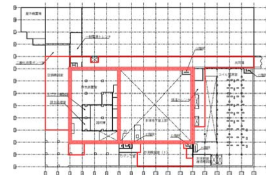
本体棟地下1階平面図
