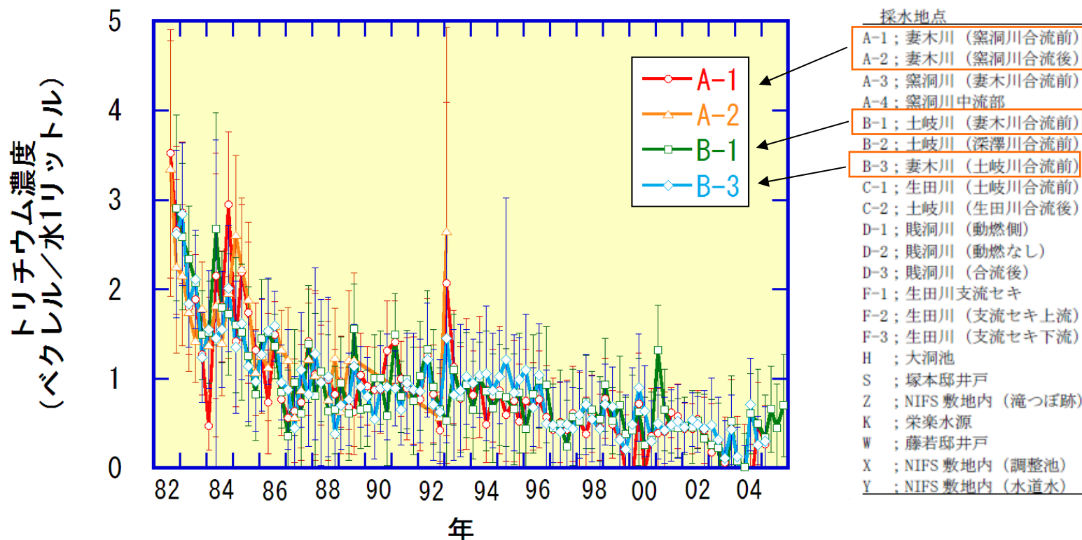
環境水トリチウム濃度の測定誤差 (20~30回計測した測定値の標準偏差を示した。)
