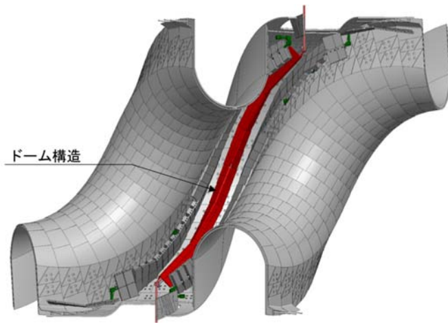
図1 LHDの閉構造ダイバータ (赤色がドームタイル)
