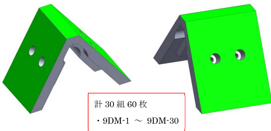
図3 タングステンコーティングの施工範囲 (緑色で示した範囲)
