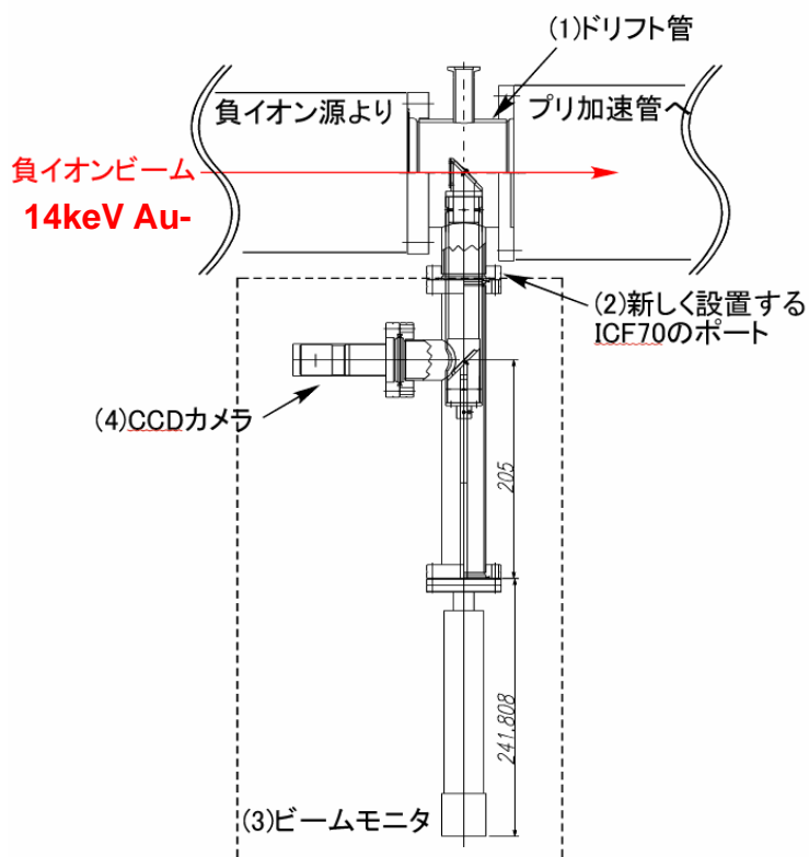
図 4-1 ビームモニターの追設内容
