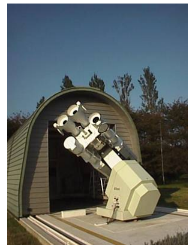
図 2. 太陽フレア望遠鏡
