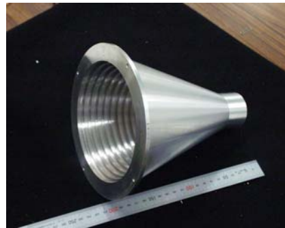
写真 8 コルゲートテーパ導波管
