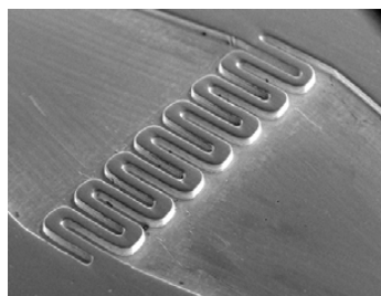
図3 マイクロミキサー用流路
