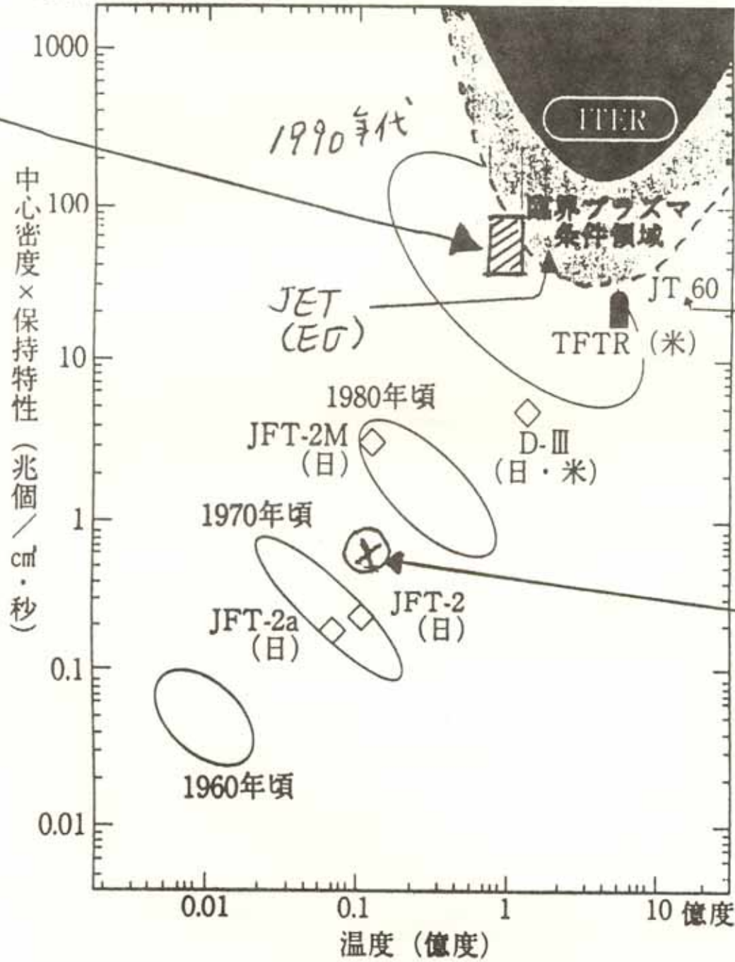
( 10^{12} ) ローソンダイアグラムとプラズマパラメータの達成値 兆個 / ( \text{cm}^3 \cdot \text{sec} )
