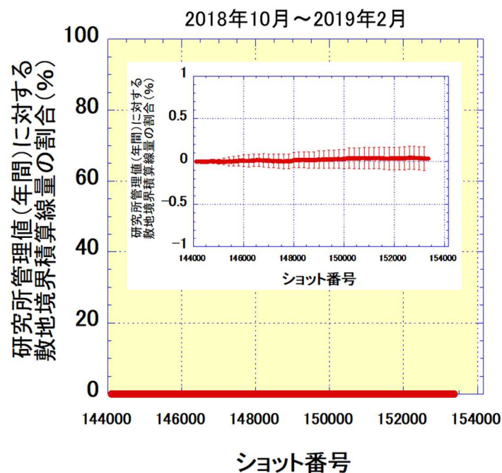
図4-2. 2 第20サイクル実験期間のLHD重水素実験開始以降のRMSAFEによる敷地境界積算線量の推移
