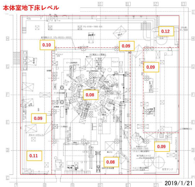
図5-4. 1 大型ヘリカル実験棟本体室（上図）、及び本体室地下（下図）における線量測定結果の例（数値の単位： \mu\text{Sv}/\text{時間} ）
