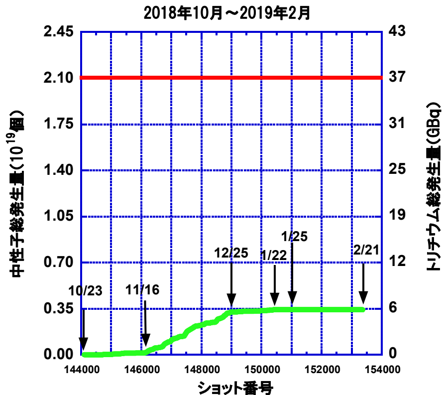
図4-1.2 第20サイクル実験期間の中性子、及びトリチウムの総発生量の推移
