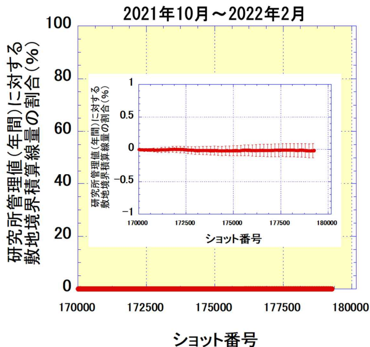
図4-2. 2 第23サイクル実験期間のLHD重水素実験開始以降のRMS AFEによる敷地境界積算線量の推移
