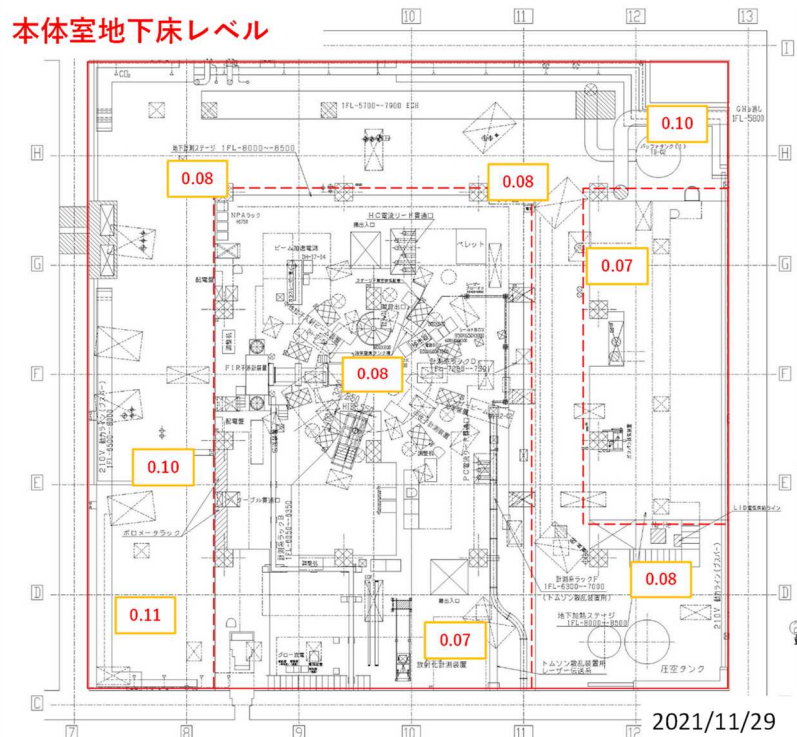
図 5-4. 1 大型ヘリカル実験棟本体室（上図）、及び本体室地下（下図）における線量測定結果の例（数値の単位： \mu S v/h）
