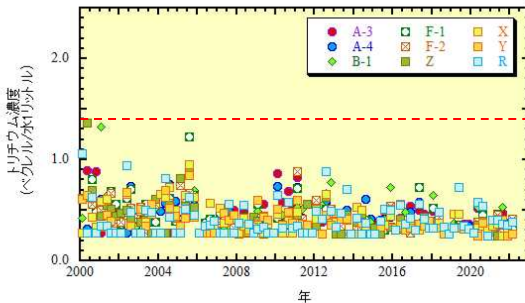
図6-1. 1 環境水の採取地点（上図）と環境水中トリチウム濃度の推移（下図） （赤点線：2000年～2016年までの変動範囲：検出下限値以下（ND）～1.4 Bq/ℓ）
