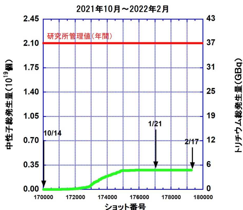
図4-1.2 第23サイクル実験期間の中性子、及びトリチウムの総発生量の推移
