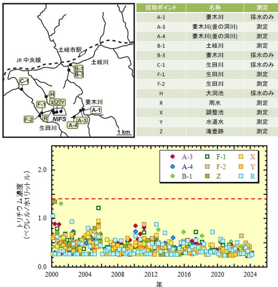
図6-1. 1 環境水の採取地点（上図）と環境水中トリチウム濃度の推移（下図）
