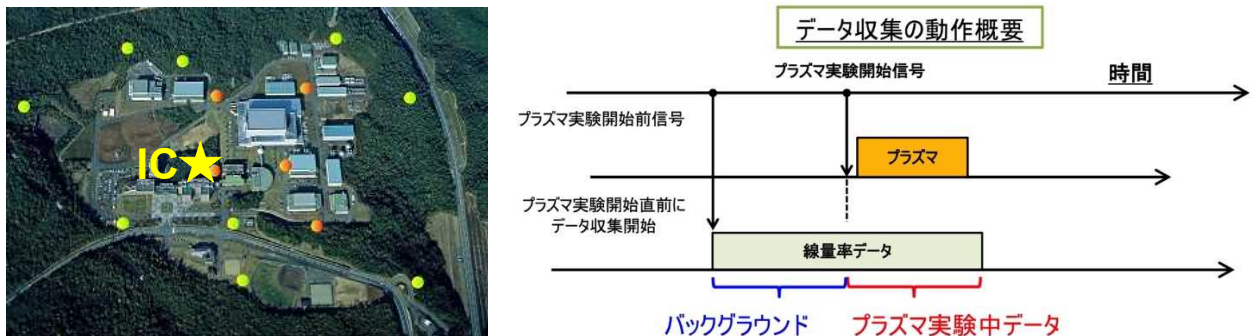
図4-1. 1 RMSAFEのICポスト地点（左図）、及びLHD実験に起因する敷地境界線量の評価のためのデータ収集システム動作概要（右図）
