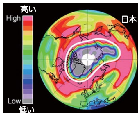
2011年3月中旬の北半球のオゾンの濃度。白い線で囲まれた領域で、オゾン層が破壊されている。 Courtesy NASA/JPL-Caltech
