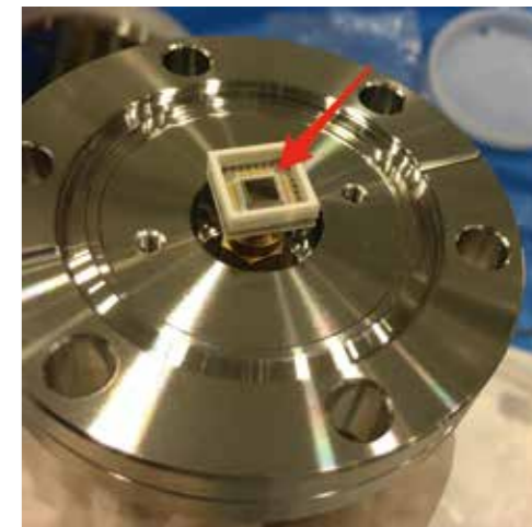
人工ダイヤモンド検出器の写真 (矢印の先の4ミリメートル四方の正方形がダイヤモンド)
