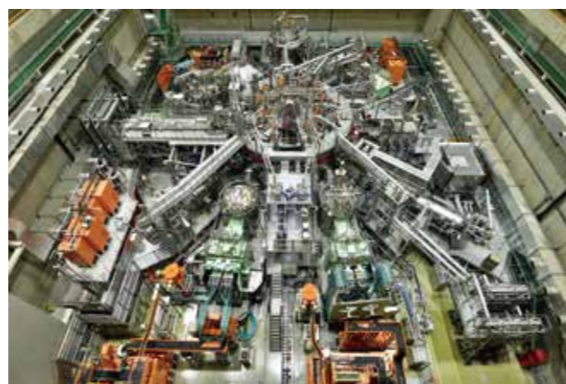
大型ヘリカル装置（LHD）全景
