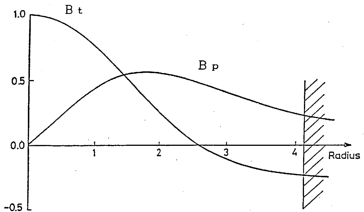
図1 逆磁場ピンチのプラズマ中の磁場分布の模式図。小半径方向の分布。
