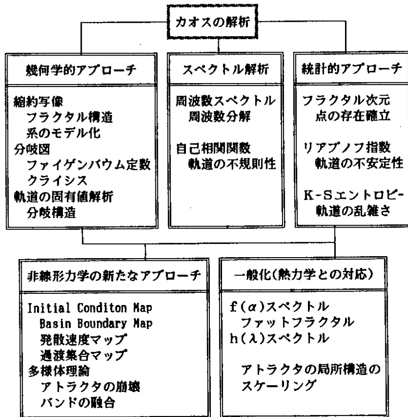
図2 カオスの研究の概略図
