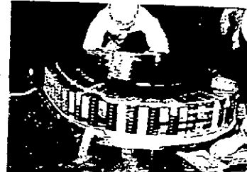
超伝導トロイダル磁場コイル(巻線作業)
