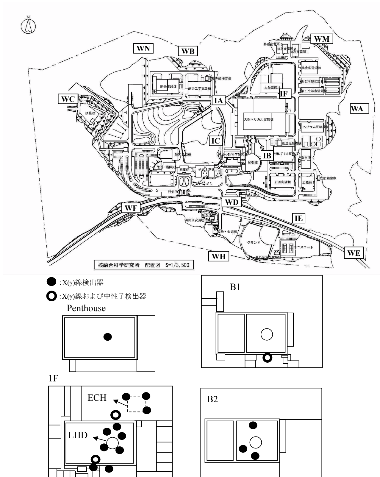
図 3-3-2 大型ヘリカル実験棟内の放射線測定器の配置
