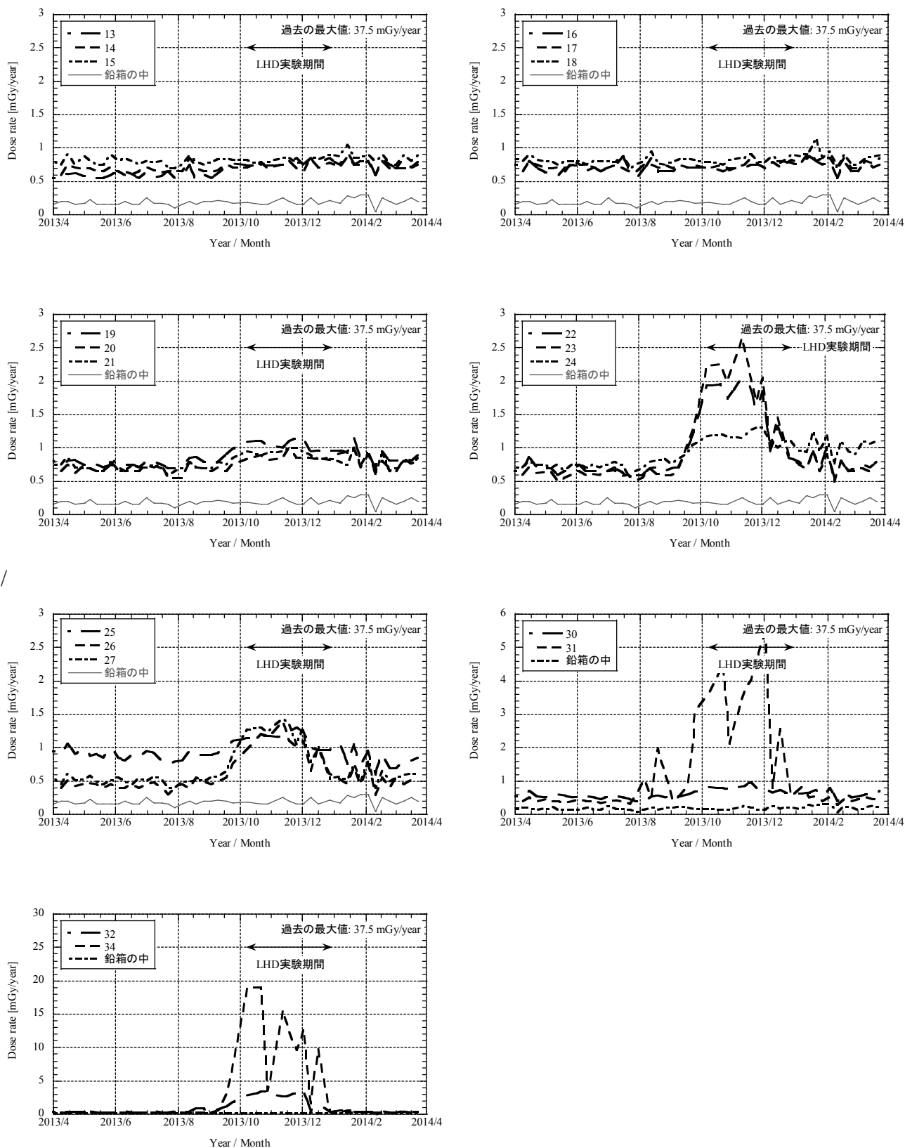
図 3-2-1 (2) 大型ヘリカル実験棟での測定結果
